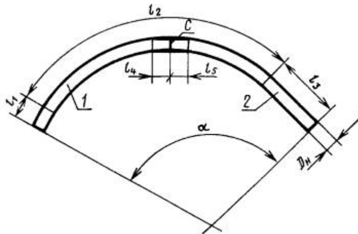
Отвод типа 3
