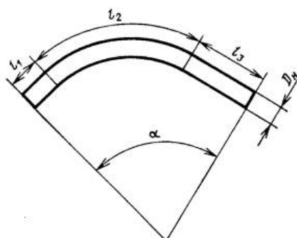
Отвод типа 1
